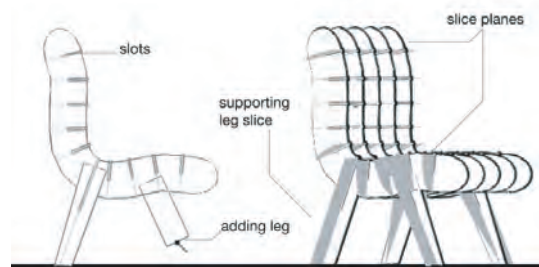
図 3. 脚の追加
